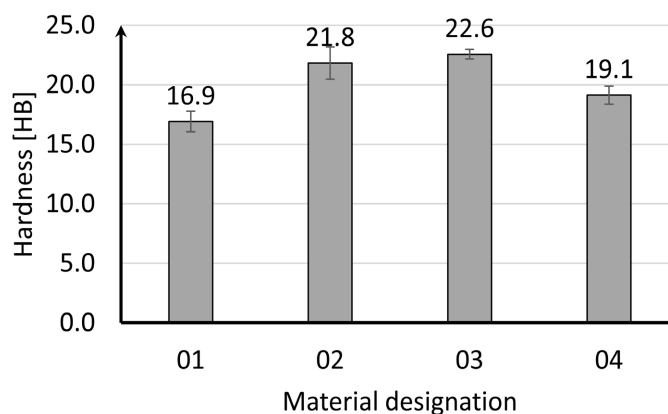
Fig. 1. Hardness of ingots
