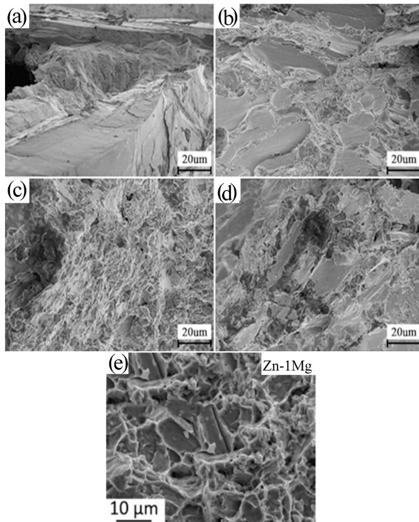
Fig. 3. SEM image of tensile fracture morphology: (a) pure zinc; (b) Zn-1Mg-1.0 wt.% Sn; (c) Zn-1Mg-2.0 wt.% Sn and (d) Zn-1Mg-5.0 wt.% Sn; (e) Zn-1Mg
